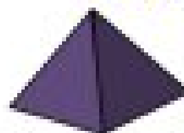
пирамида
