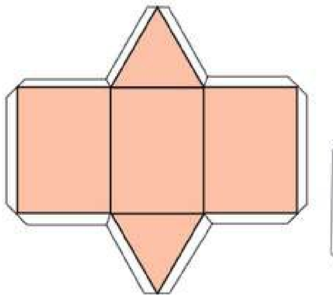
Треугольная призма
