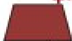
четырёхугольник
